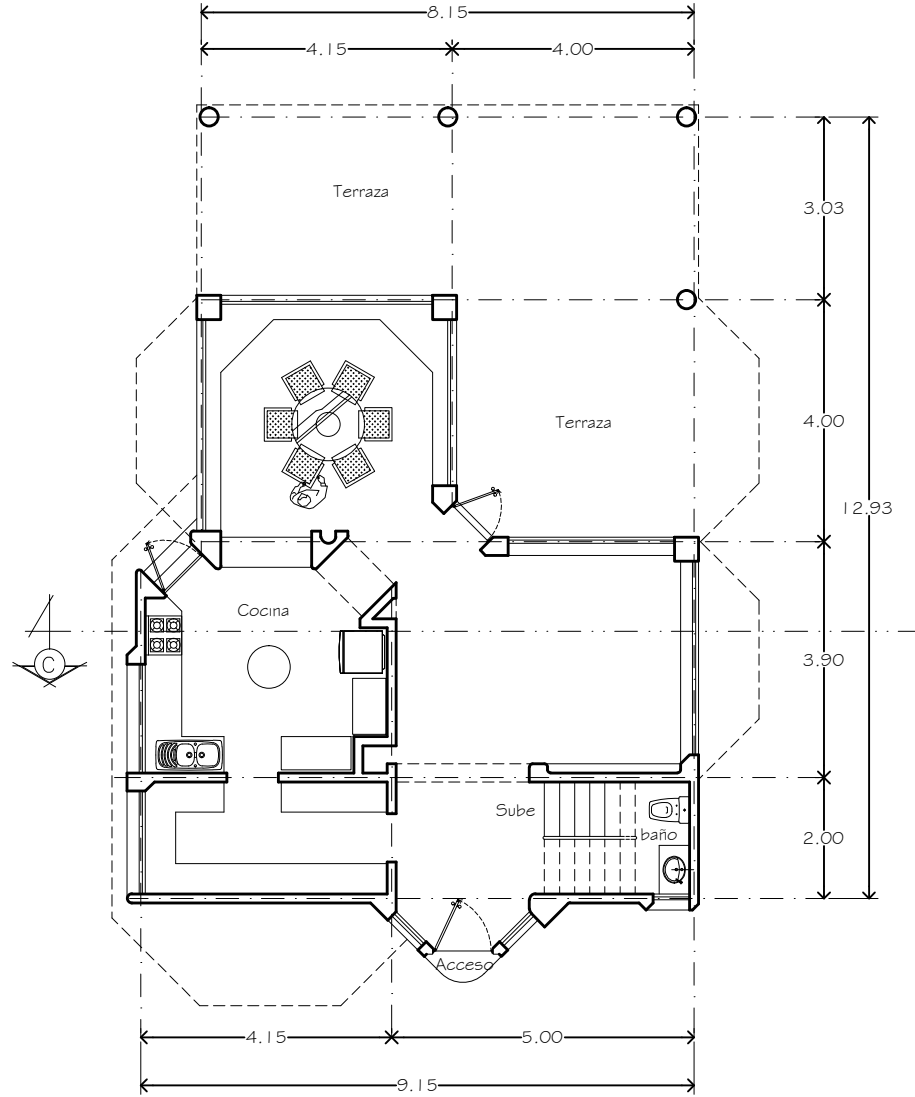
Planta Baja _____ esc. 1 : 75
