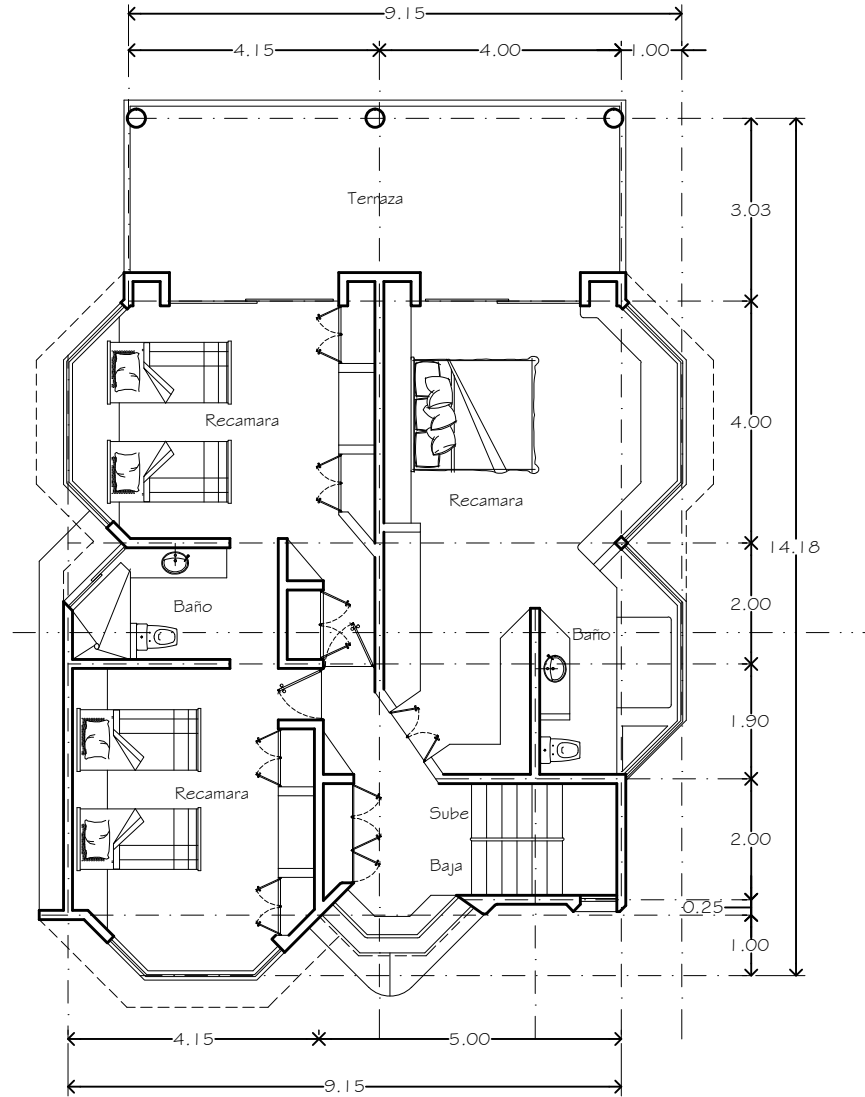
Planta 1er Nivel _____ esc. 1 : 75
