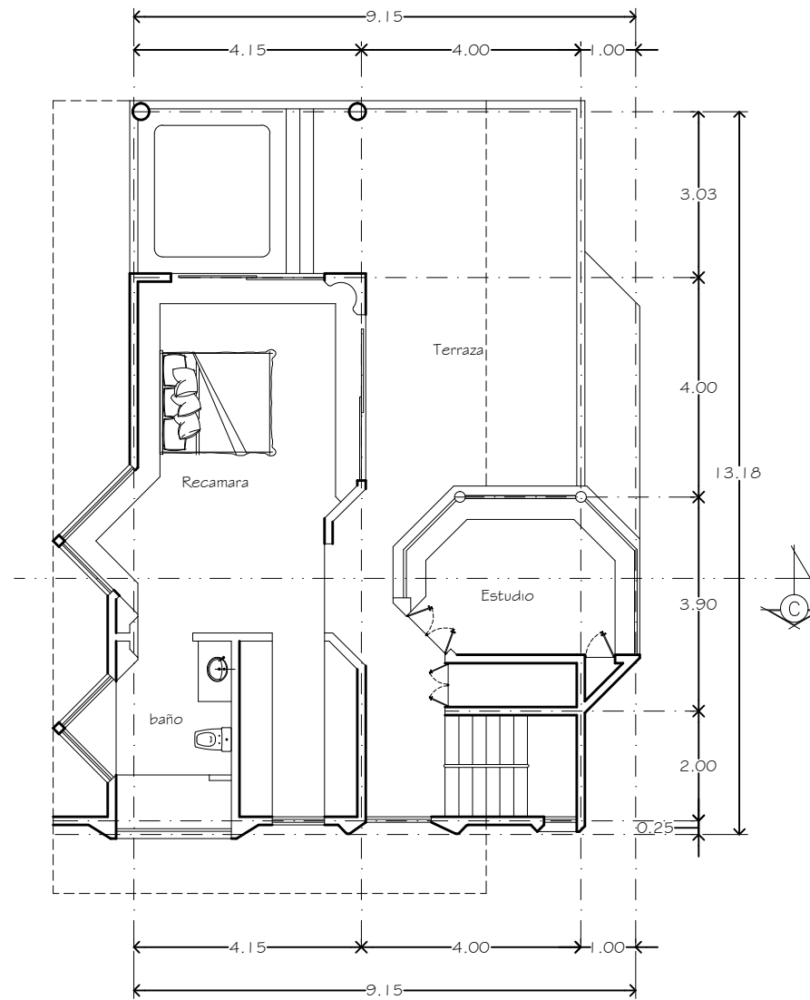
Planta 2do Nivel _____ esc. 1 : 75
