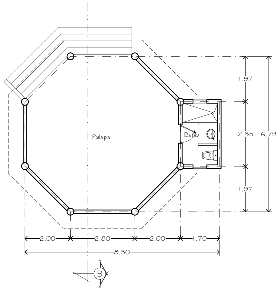
Planta Nivel Alberca _____ esc. 1 : 75
